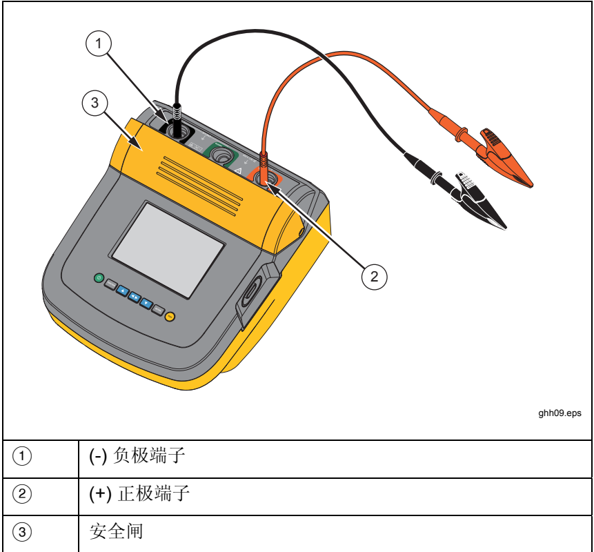
图 9. 测试导线连接
